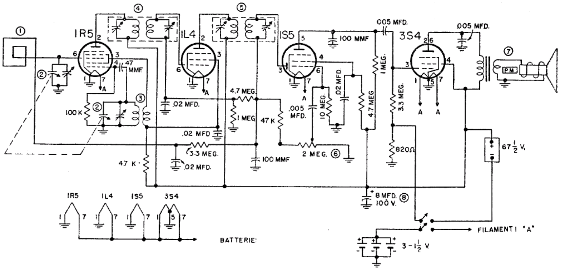
- Schema di portatile "40 ore" americano (Garod mod. 4B1).
